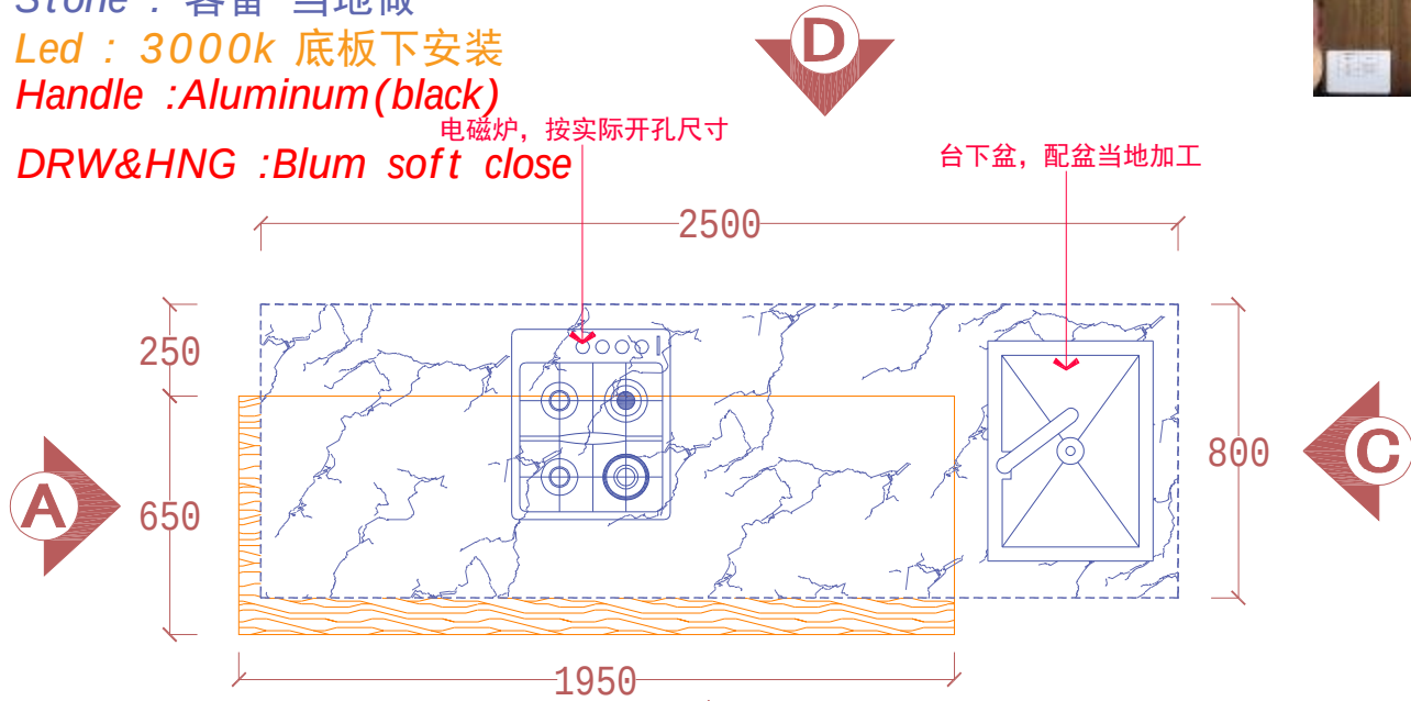
外观视图
