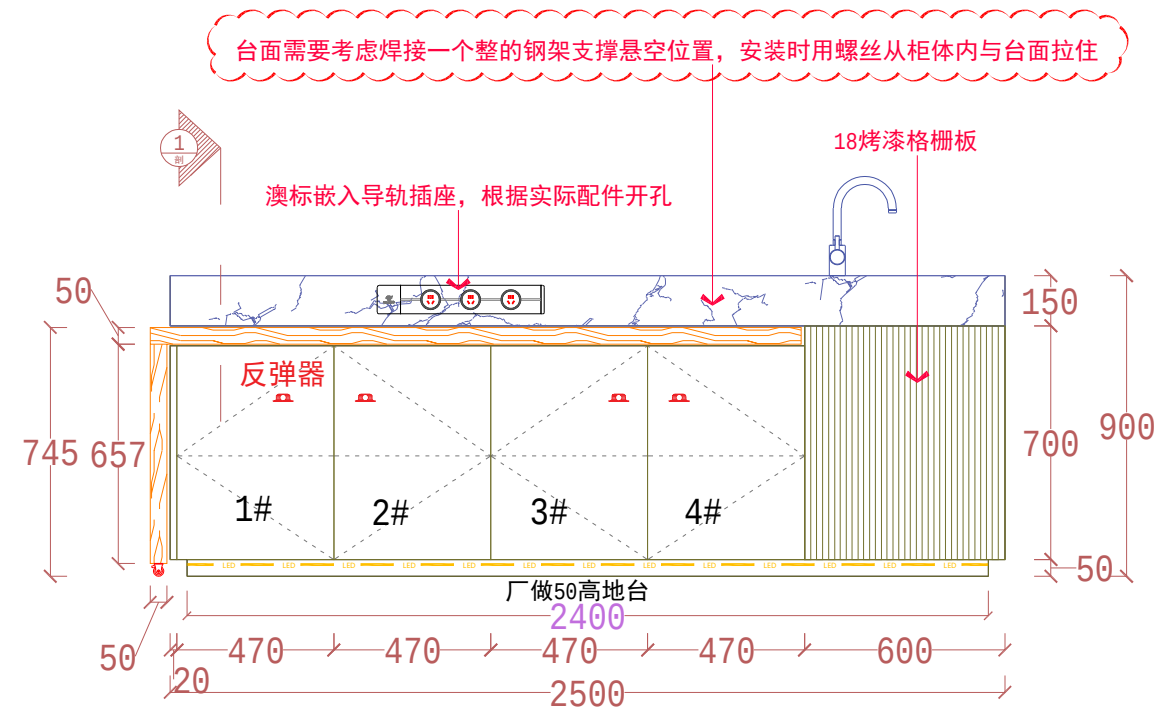
ELEVATION B
