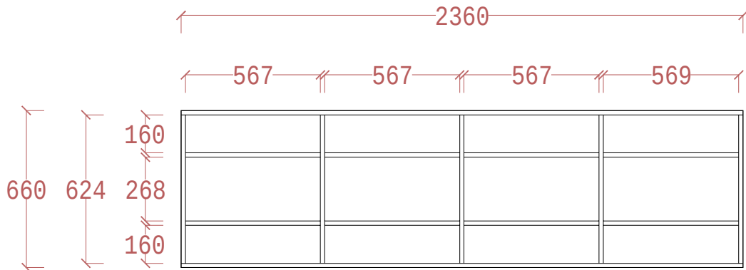
地台平面图（柜体板）
