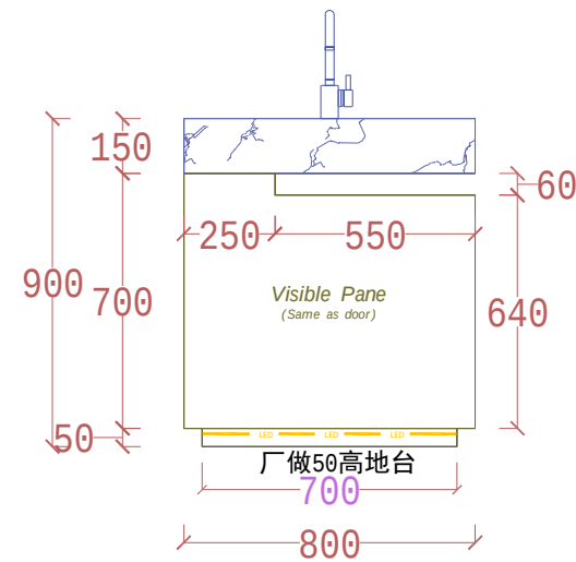
ELEVATION A
