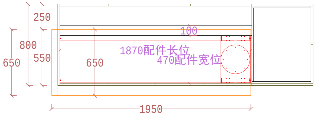
配件视图
