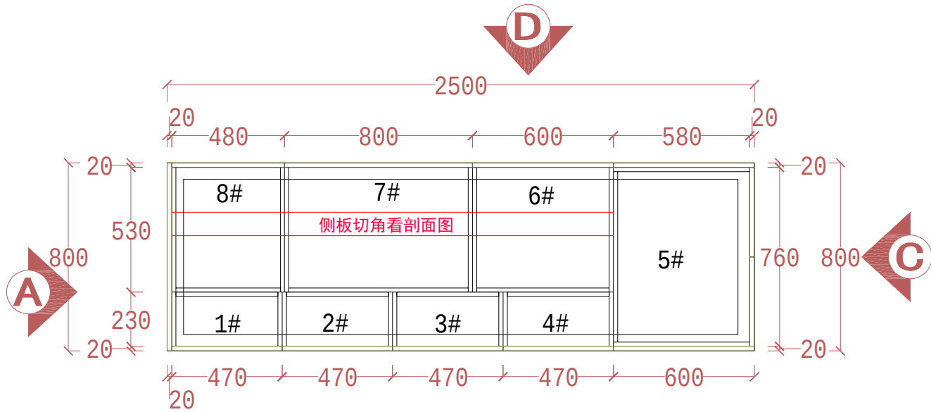
外观视图
